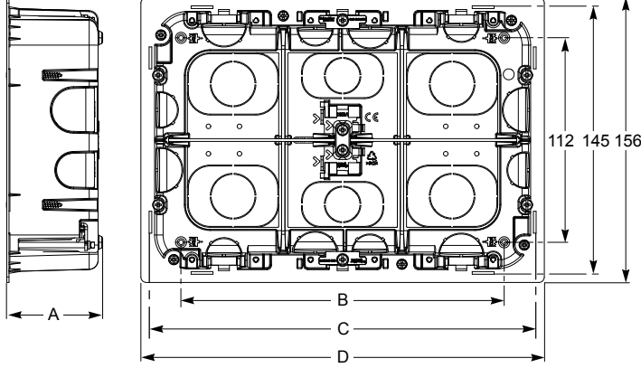
Yatay sıva altı ortalama kasalar
