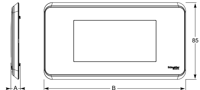
Unica Pro
