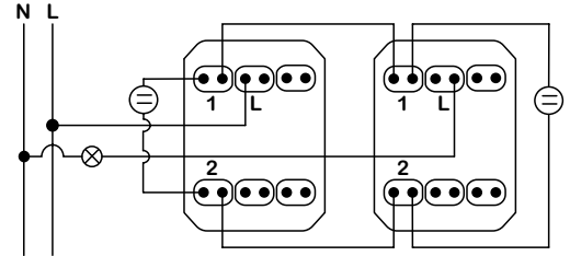
2 modül - Işıklı vavien
