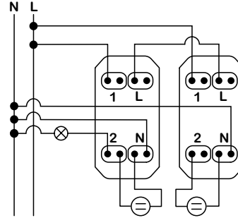
1 modül - Gösterge lambalı ve nötr bağlantılı 2 vavien
