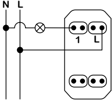
1 modül - Anahtar Liht buton
