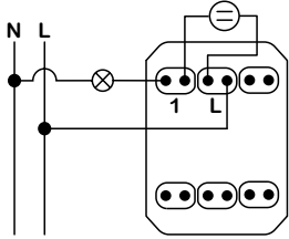
2 modül - Işıklı anahtar
