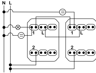
2 modül - Gösterge lambalı 2 vavien
