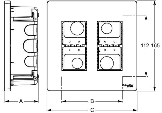
Dikey sıva altı çalışma istasyonu kasaları
