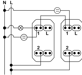
1 modül - Gösterge lambalı 2 vavien
