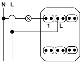
2 modül - Anahtar Liht buton
