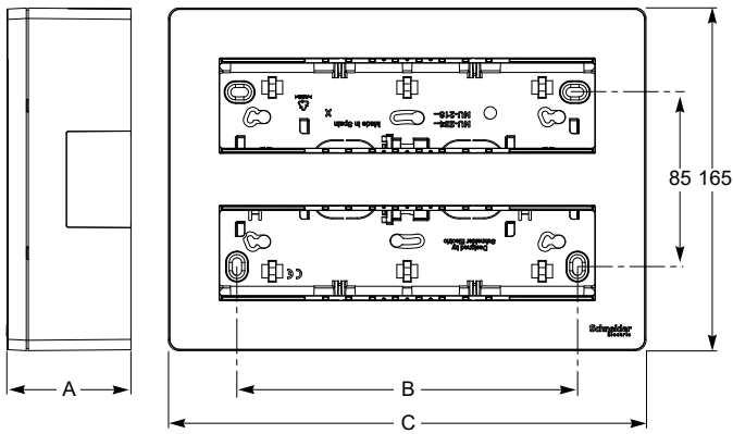
Yatay sıva üstü çalışma istasyonu kasaları
