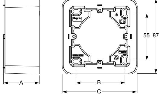
Unica Pro sıva üstü kasalar
