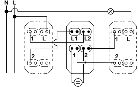
1 modül - Işıklı 2 vavien + 1 permütatör
