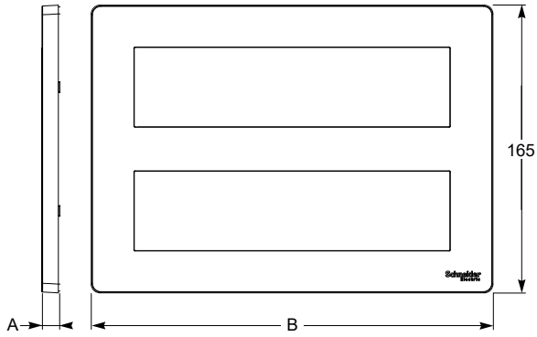
Yatay çerçeve
