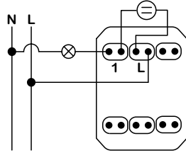
2 modül - Işıklı liht buton
