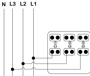
3 kutuplu anahtar
