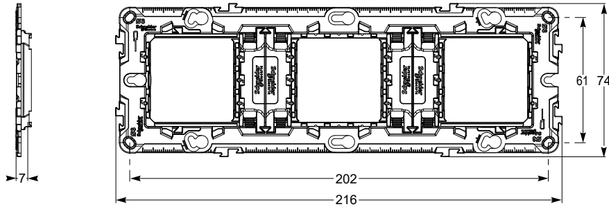
NU7006C
