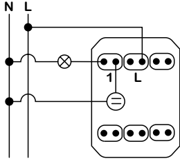
1 modül - Gösterge lambalı anahtar
