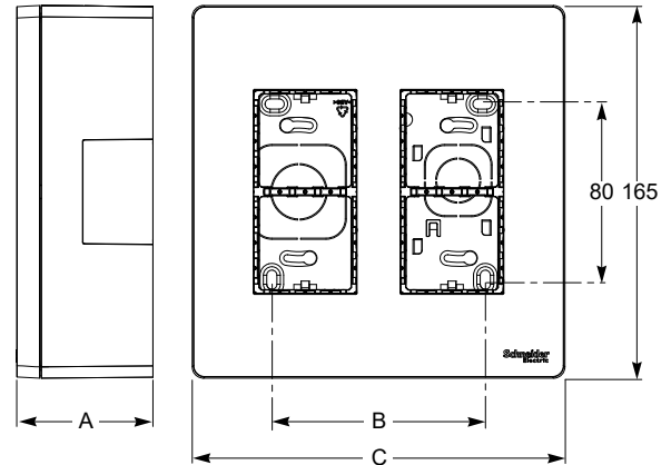
Dikey sıva üstü çalışma istasyonu kasaları
