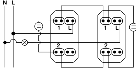
1 modül - Işıklı 2 vavien
