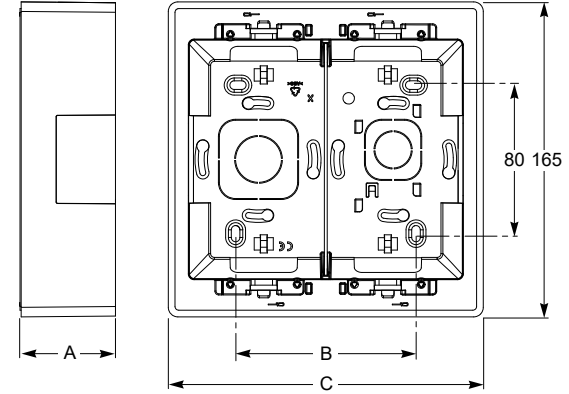
Dikey ortalama kasalar
