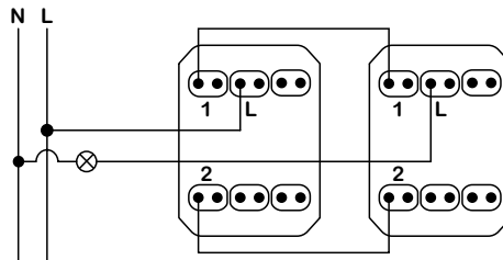
2 modül - Vavien
