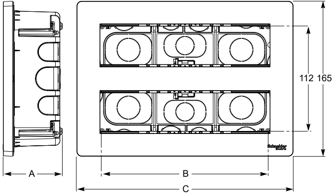
Yatay sıva altı çalışma istasyonu kasaları
