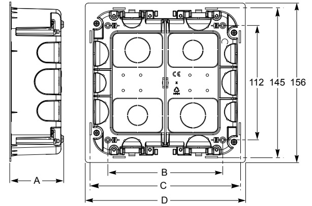
Dikey sıva altı ortalama kasalar
