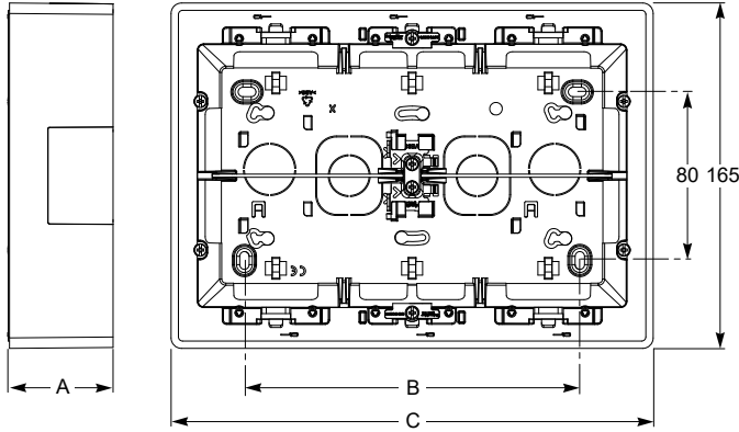
Yatay ortalama kasalar
