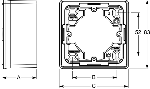
Unica Studio sıva üstü kasalar
