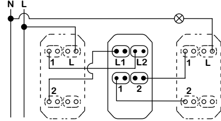
1 modül - 2 vavien + 1 permütatör
