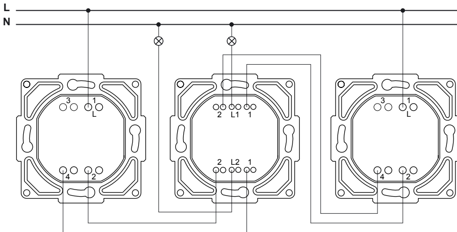
2 vavien anahtar + farklı iki yükte çalışan 1 ikili vavien
