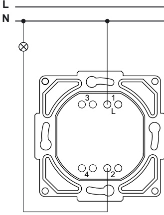
Işıklı anahtar
