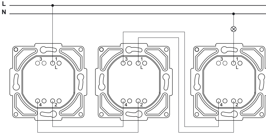
2 vavien + 1 permütatör
