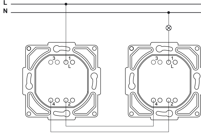
2 ışıklı vavien
